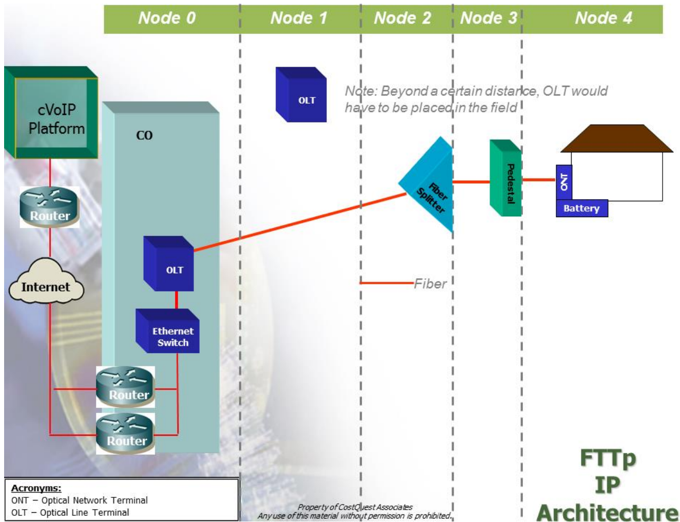
Figure 10--FTTP topology
